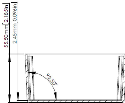
SECTION A-A SCALE 2 : 3
