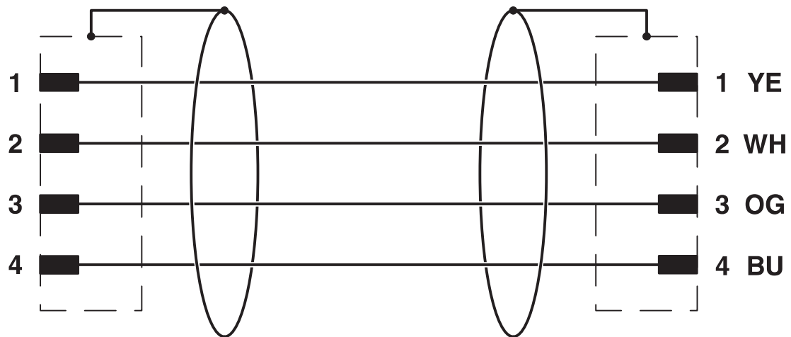
M8针式连接器触点分配
