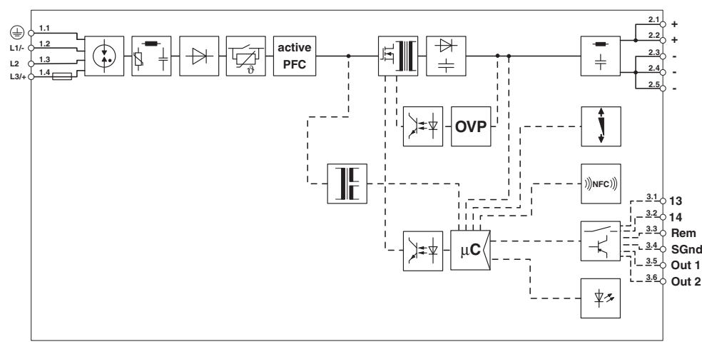
结构框图
