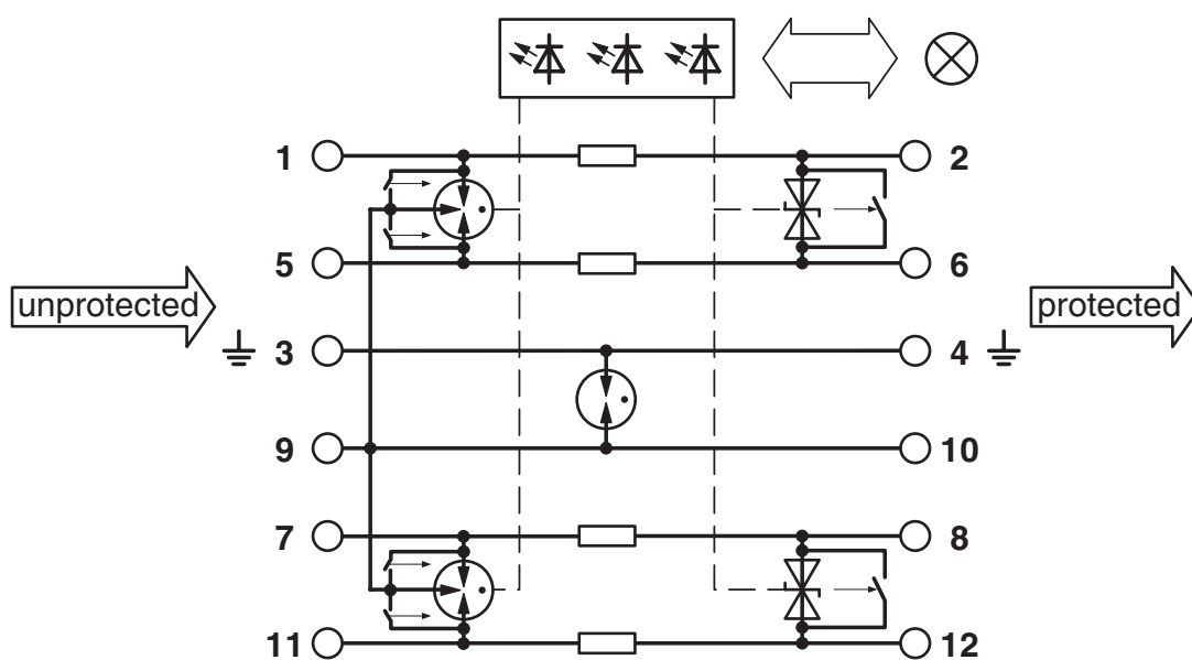
电路图
