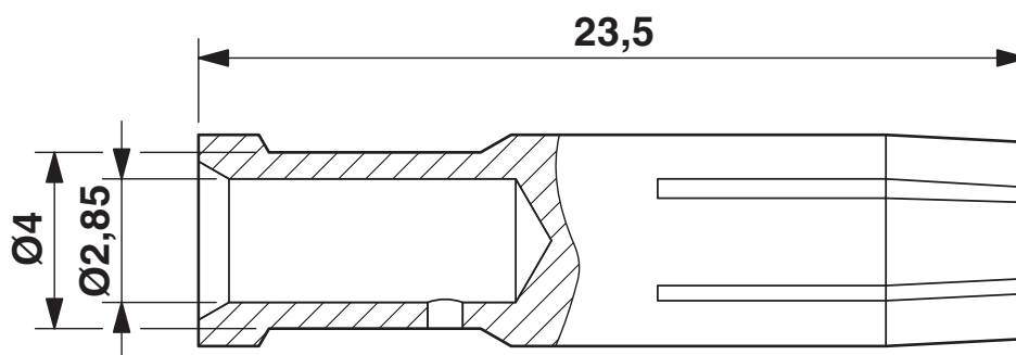
尺寸图
