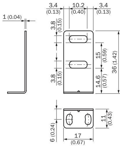
尺寸图 (尺寸单位: mm)
