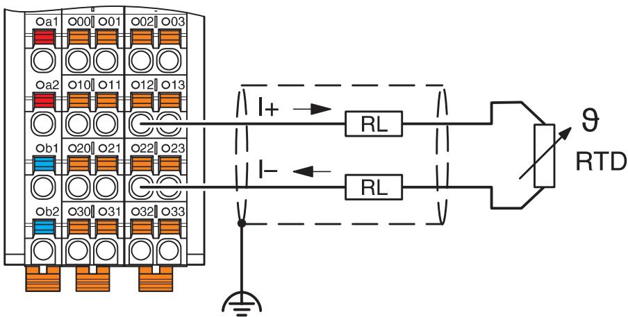
接线图
