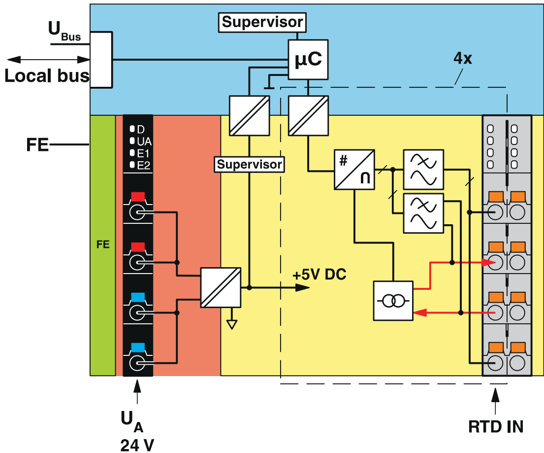
结构框图
