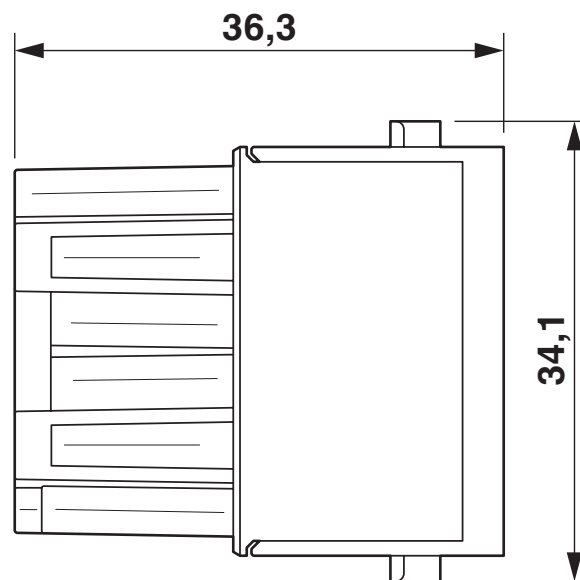
尺寸图
