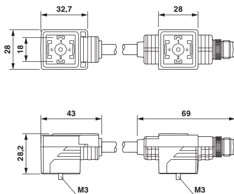
外形寸法
