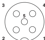
配線図
