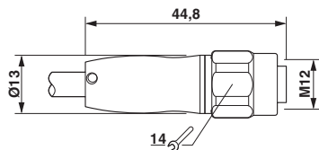
外形寸法
