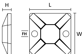
Festesokkel MB3, MB4, MB5
