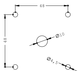
Bohrbild Tuer
