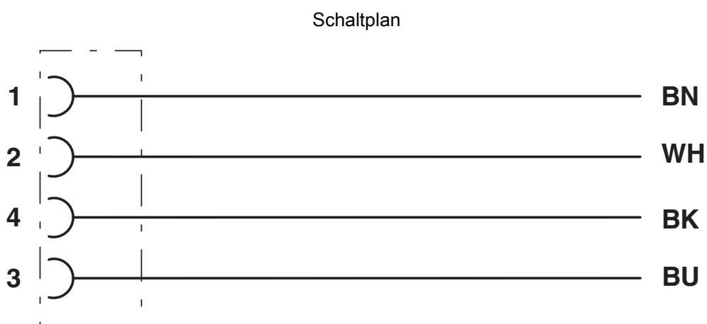
Kontaktbelegung des M12-Steckers
