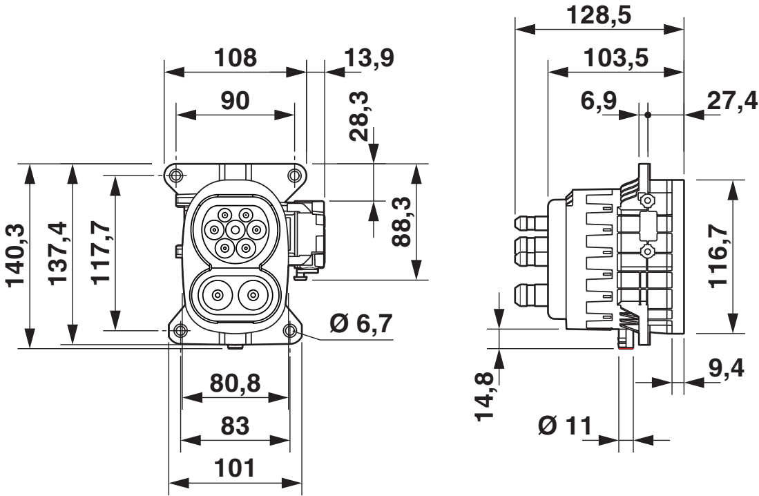
尺寸图
