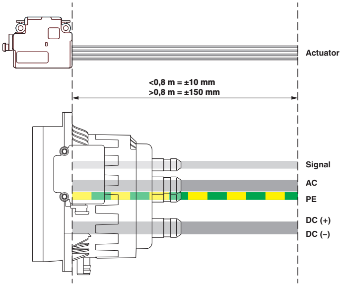
尺寸图
