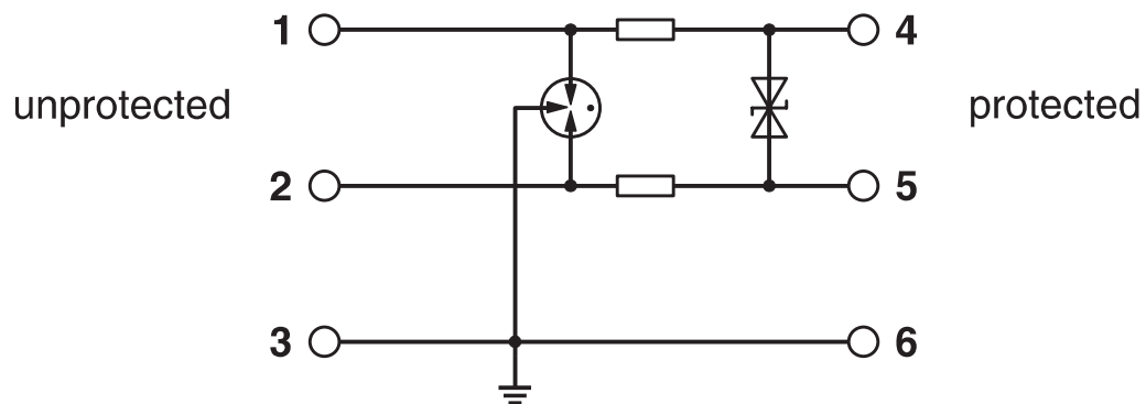
电路图
