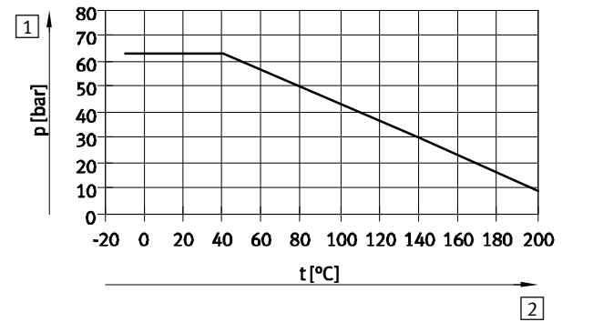
1 Druck p [bar] 2 Mediumtemperatur t [°C] Fig. 5 Druck – Temperatur-Diagramm
