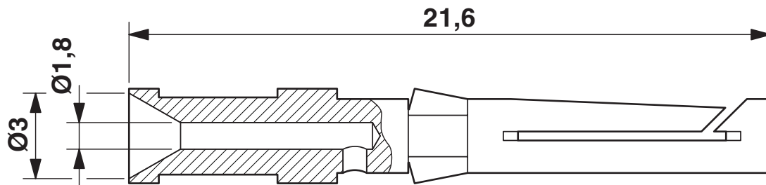
尺寸图
