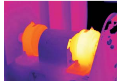
Überhitzter Lagerdeckel
