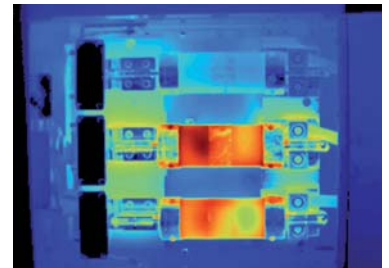
Unsymmetrische Last in einer Dreiphasen-Schaltanlage
