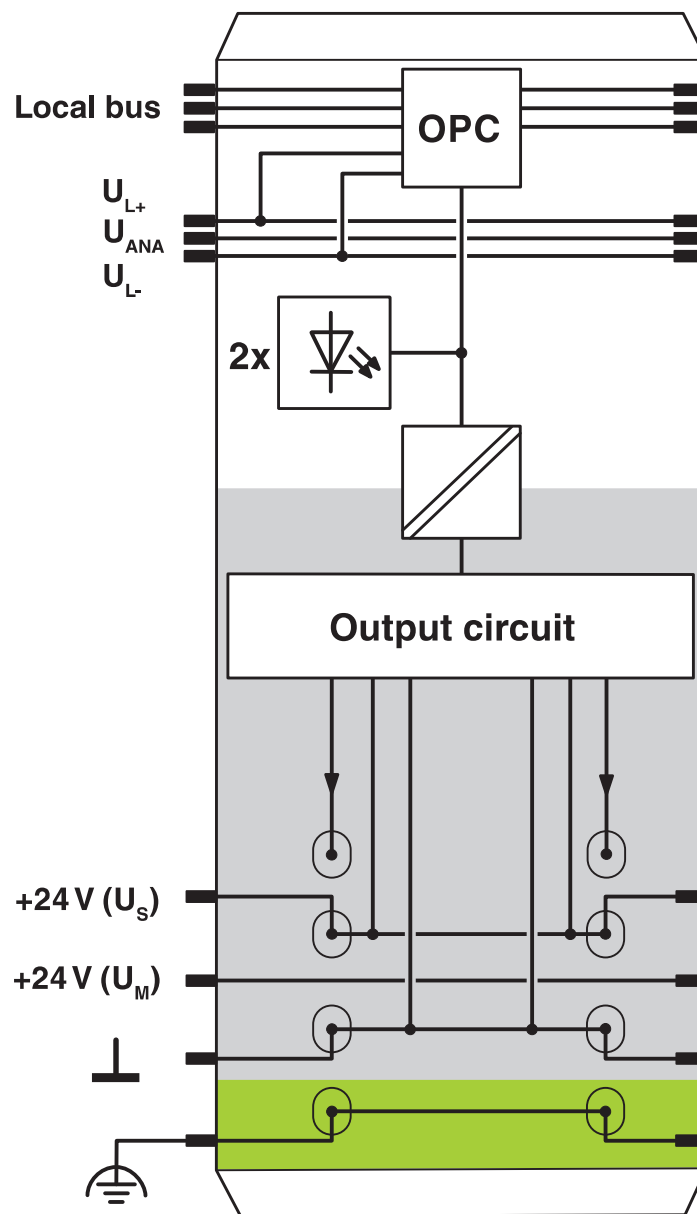
结构框图
