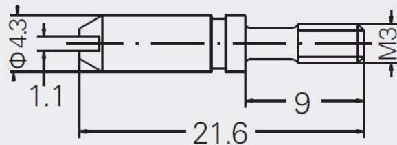
Modular guide pin
