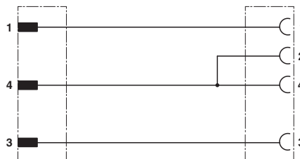
回路図
