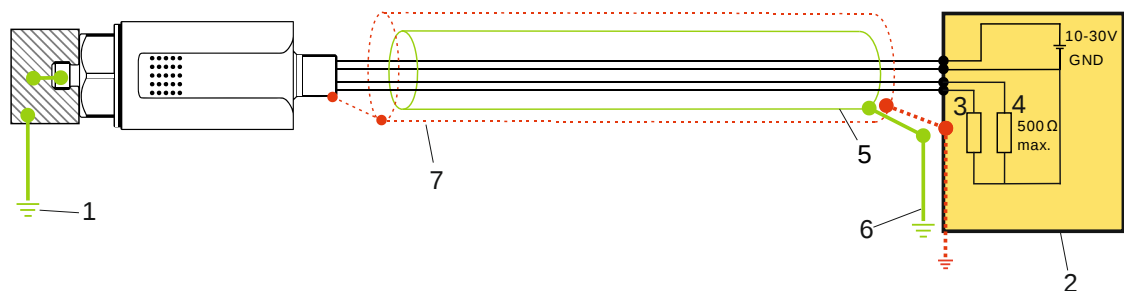
Fig. 10: Standardjordningskoncept
