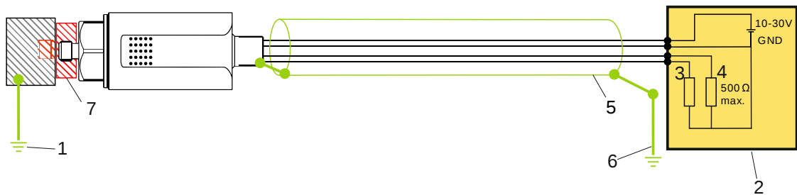
Fig. 11: Alternativt jordningskoncept
