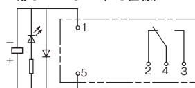
形G2R-1-SND (DC仕様)
