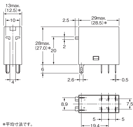
形G2R-2-SN (DC仕様)
