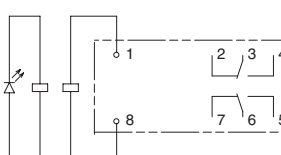
端子配置/内部接続図 (BOTTOM VIEW)
