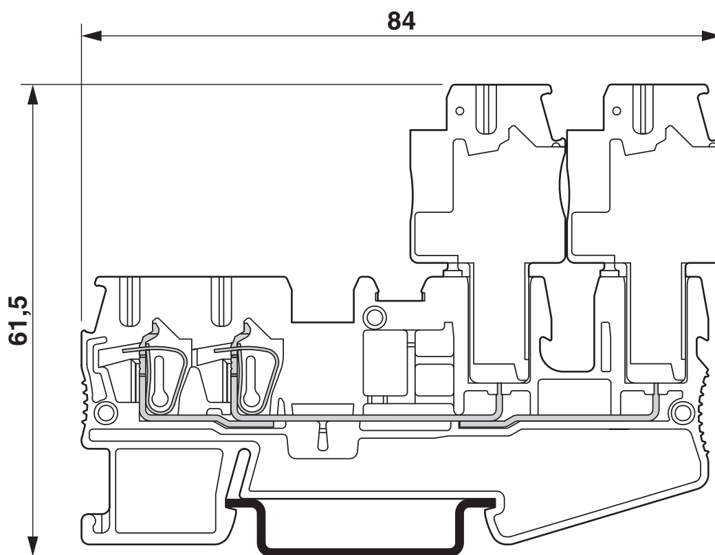
尺寸图
