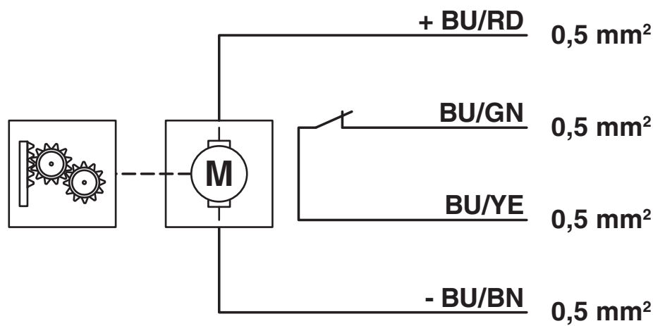
结构框图
