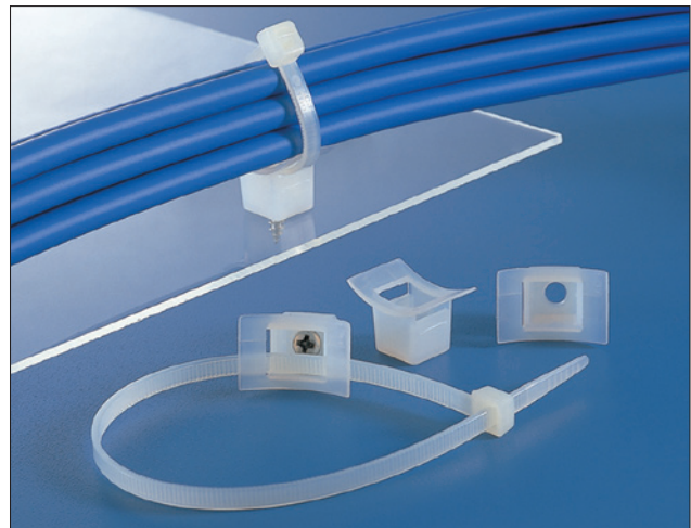
Bevestigingszadel LKC-serie.
