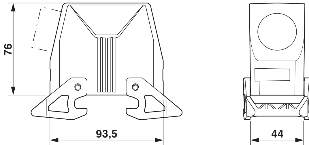
尺寸图
