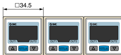
Schalttafelöffnung
