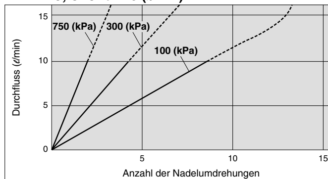
PFM710, 510 für 10 (l/min)
