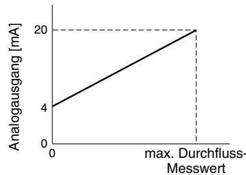
analoger Stromausgang (4 bis 20 mA)
