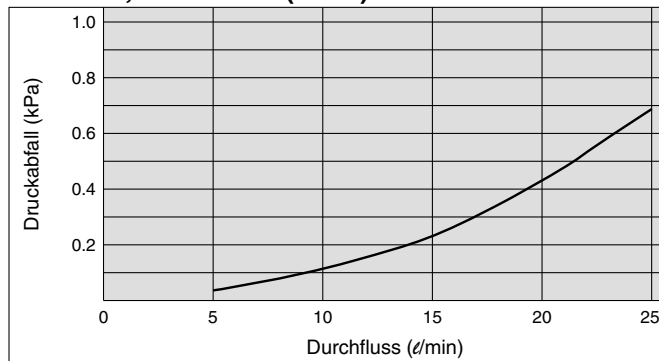
PFM725, 525 für 25 (l/min)
