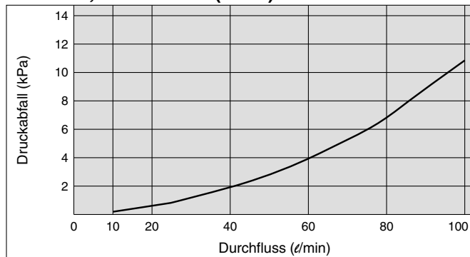
PFM711, 511 für 100 (l/min)
