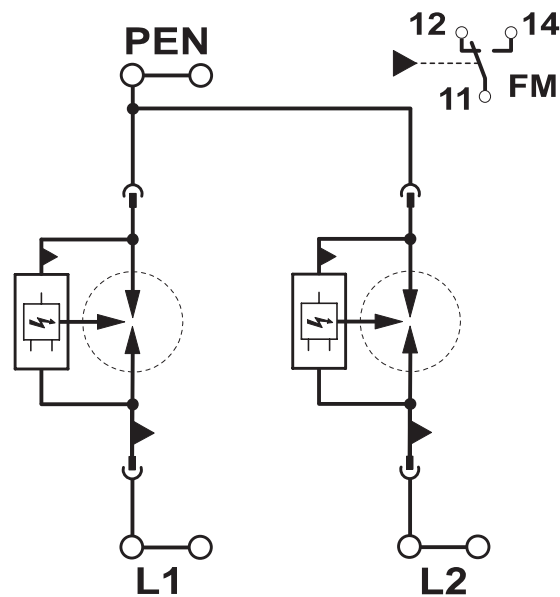
电路图
