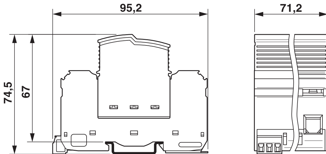
尺寸图
