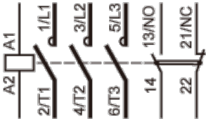
1NO+1NC(LANN11)
