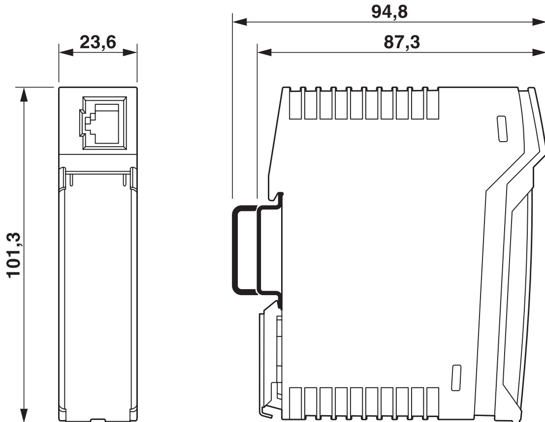
尺寸图
