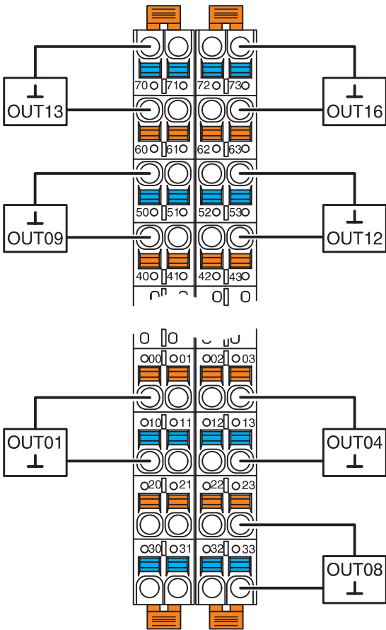
接线图
