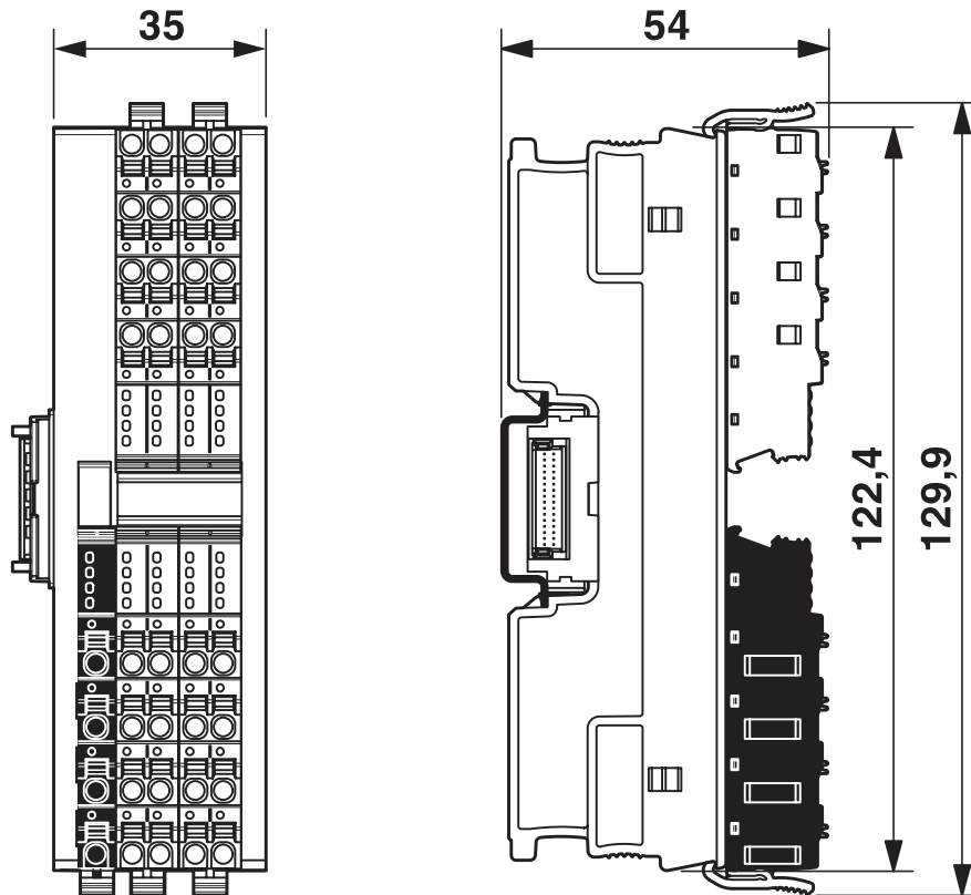
尺寸图
