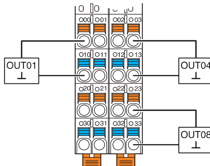
接线图
