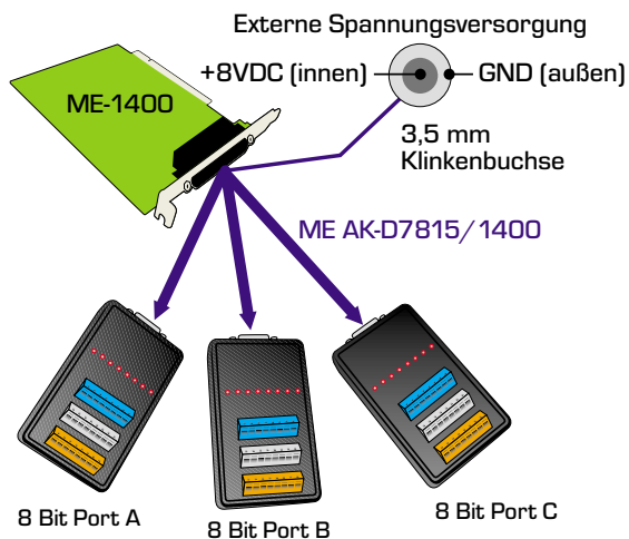
Abb. 3: Anschluß ME-1400/A/B
