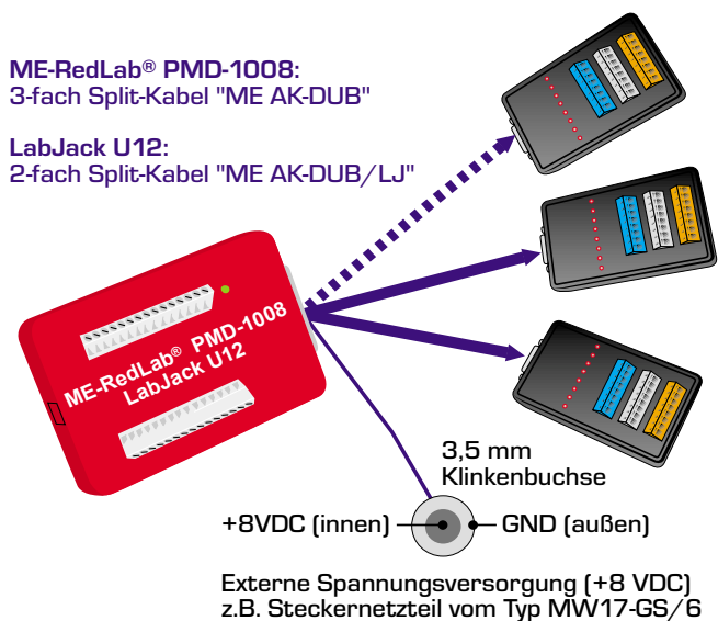
Abb. 2: Anschluß USB-Messboxen
