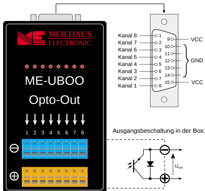
Abb. 1: Anschlußbelegung
