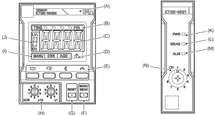
メインユニット 形K7GE-MGM
