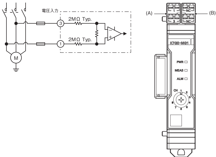
プローブユニット 形K7GE-MG1
