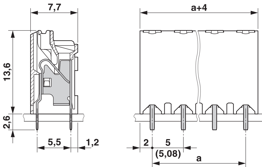
尺寸图
