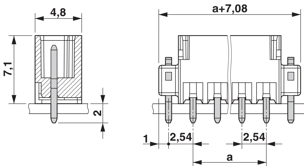
尺寸图
