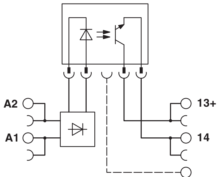
电路图
