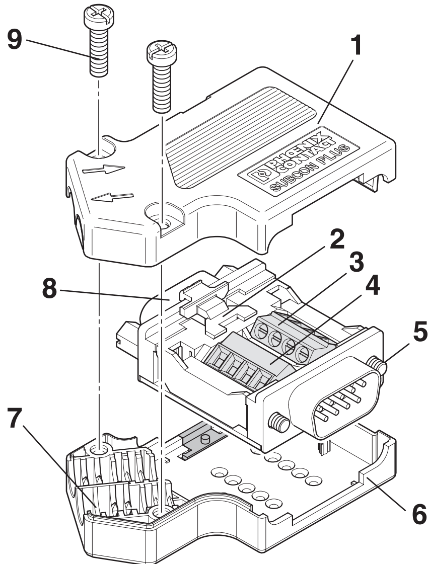
Schemazeichnung
