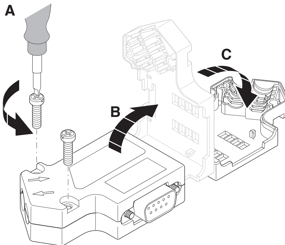
Schemazeichnung
