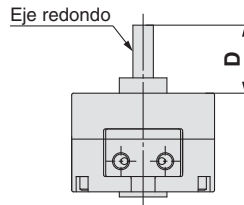
Eje simple/CRB2□T
