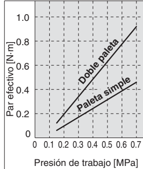
Tamaño 30
