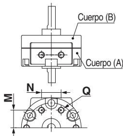
La figura superior muestra la serie CRB2.
