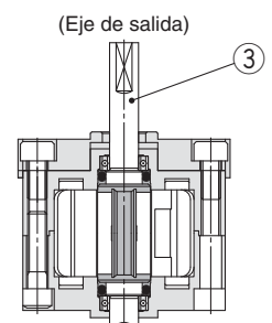
Modelo de eje doble
