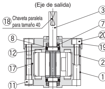
Modelo de eje simple
