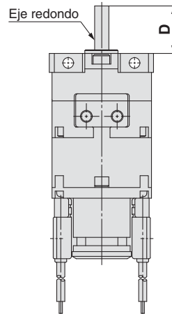
Eje doble/CRBU2JU
