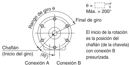
La figura superior muestra la serie CRB2. (Visto desde el lado del eje largo)
