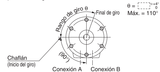
El inicio de la rotación es la posición del chaflán (de la chaveta) con conexión B presurizada. La figura superior muestra la serie CRB2. (Visto desde el lado del eje largo)
