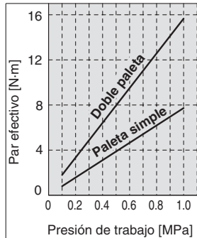
Tamaño 40
