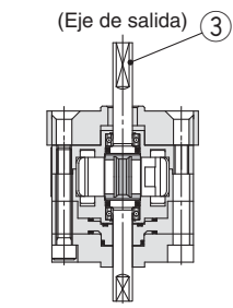
Modelo de eje doble
