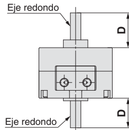
Eje doble/CRB2□JU
