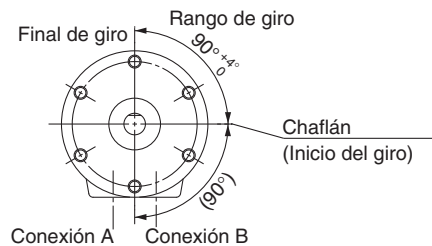
El inicio de la rotación es la posición del chaflán (de la chaveta) con conexión A presurizada. La figura superior muestra la serie CRB2. (Visto desde el lado del eje largo)
