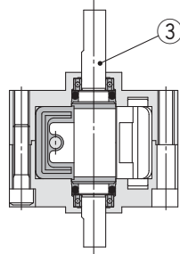
Modelo de eje doble
