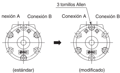
La figura superior muestra la serie CRB2. (Visto desde el lado del eje corto)
