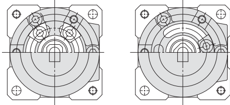
Paleta simple
