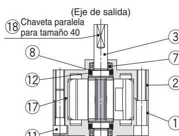
Modelo de eje simple
