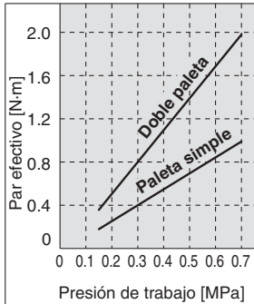
Tamaño 20
