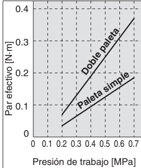
Tamaño 20
