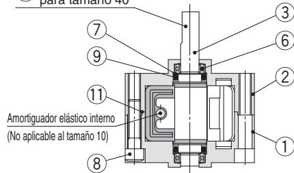
Modelo de eje simple
