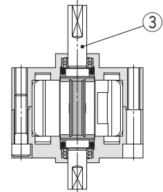
Modelo de eje doble
