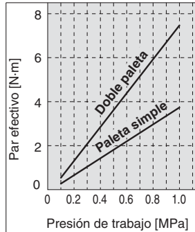
Tamaño 30
