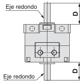
Eje doble/CRBU2K
