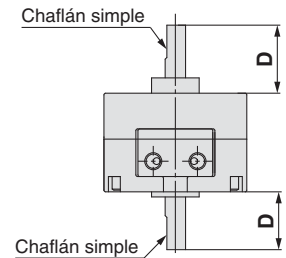
Eje simple/CRB2□Y
