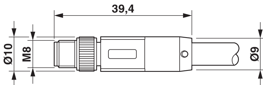
尺寸图
