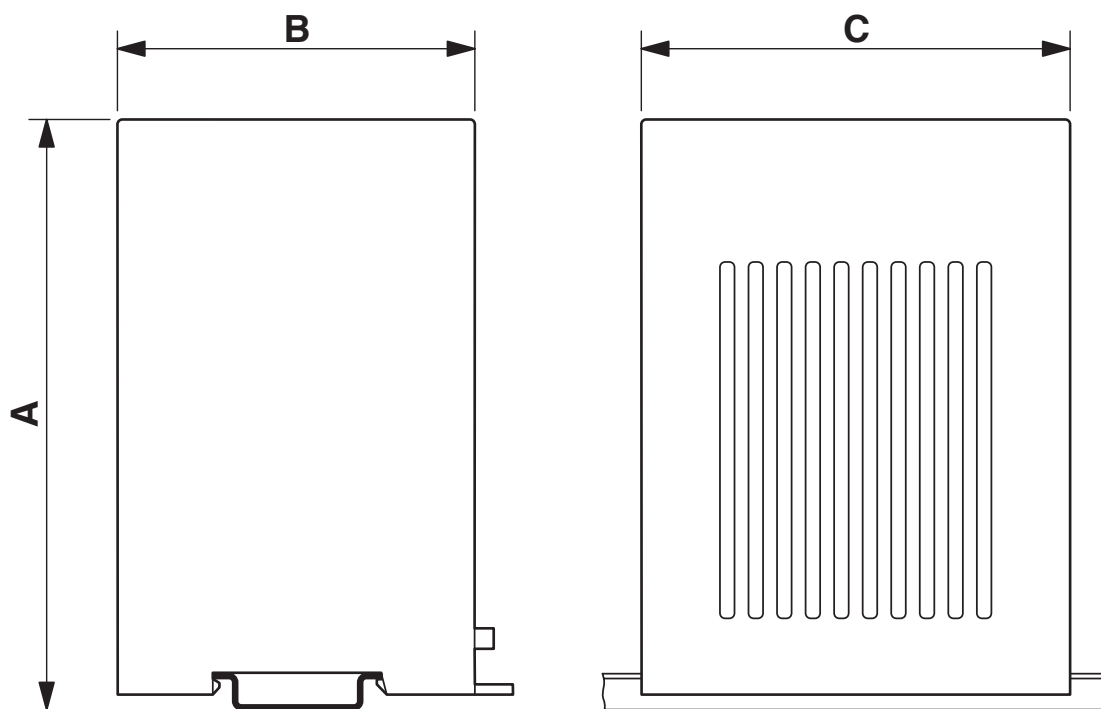
尺寸图
