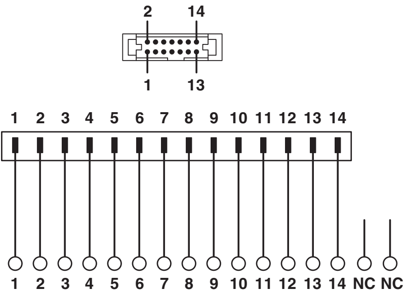
电路图
