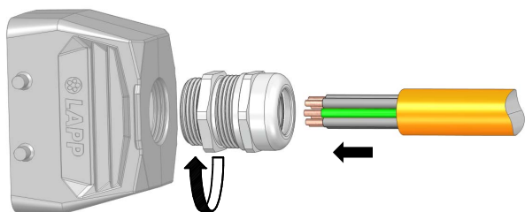
Kabelverschraubung anschliessen Mount a cable gland
