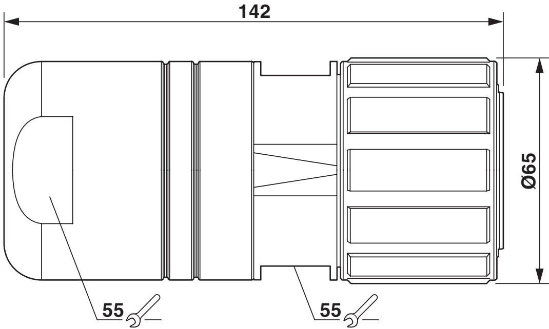
尺寸图
