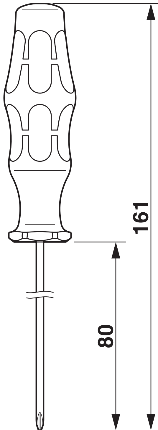
Maßzeichnung
