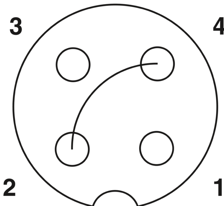
Rysunek schematyczny
