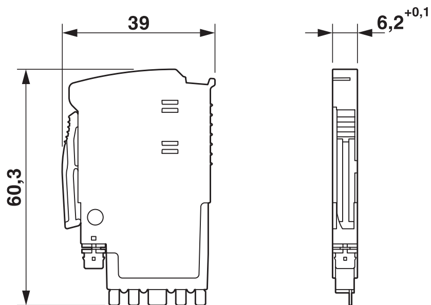
尺寸图
