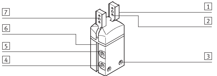
Fig. 1: Bedienteile und Anschlüsse
