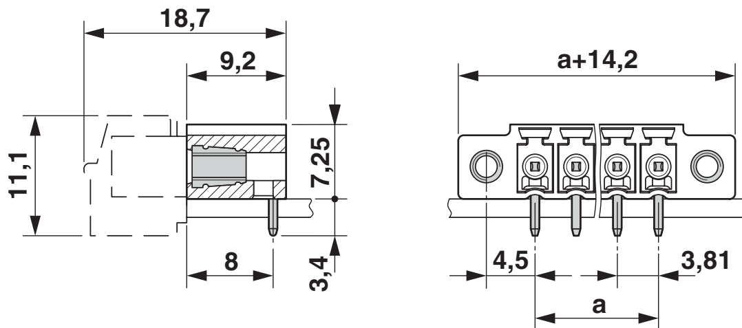
尺寸图
