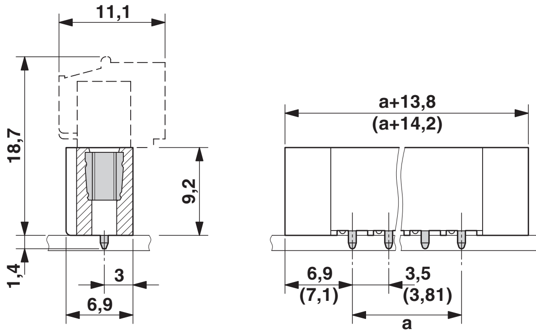
尺寸图
